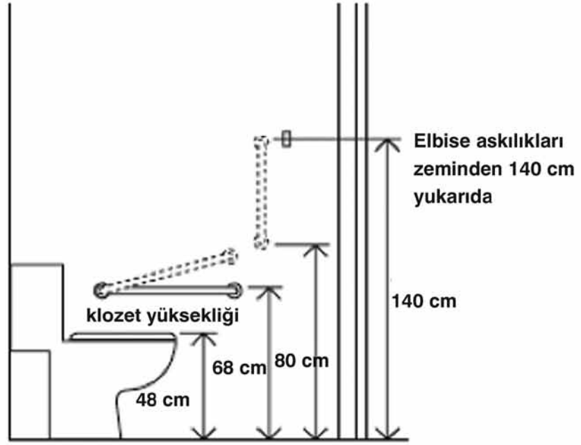
Tuvalet yerleşiminde kabul edilebilir yükseklikler
