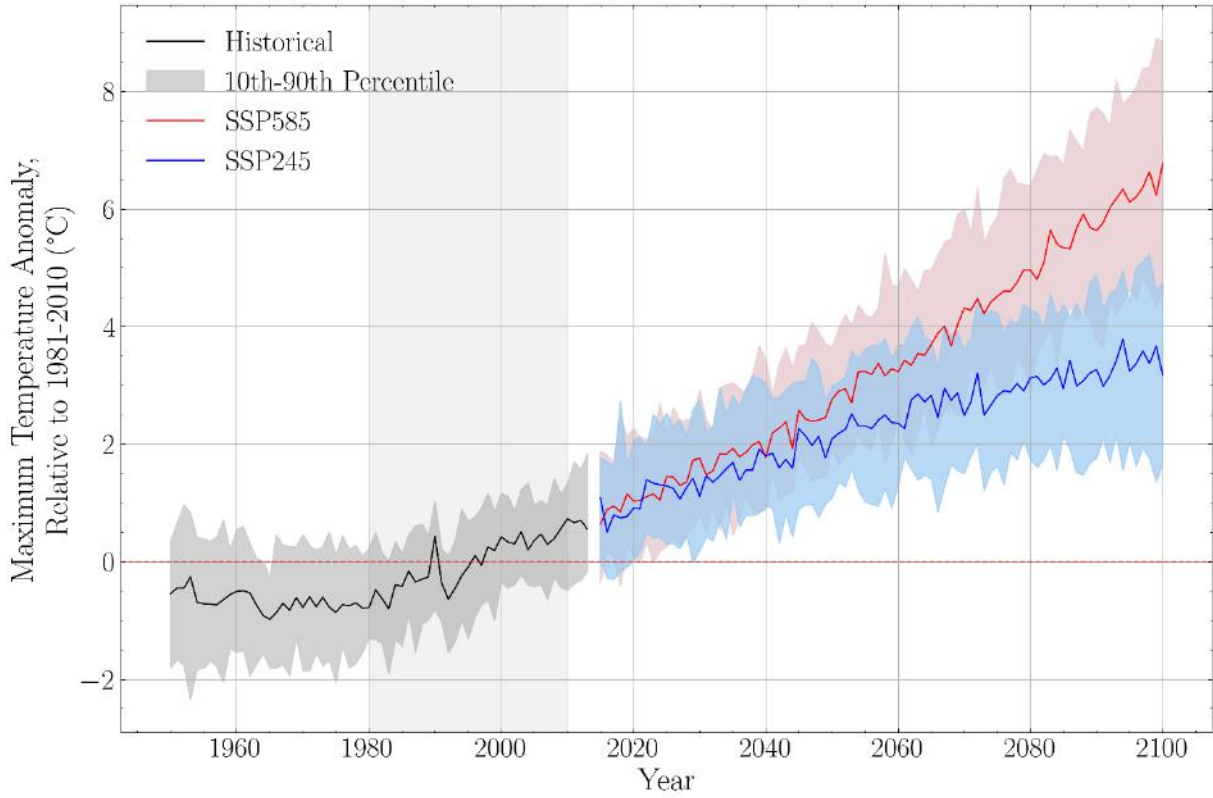
Şekil 5.4 1981-2010 Dönemine Göre Maksimum Sıcaklık Anomalisi
