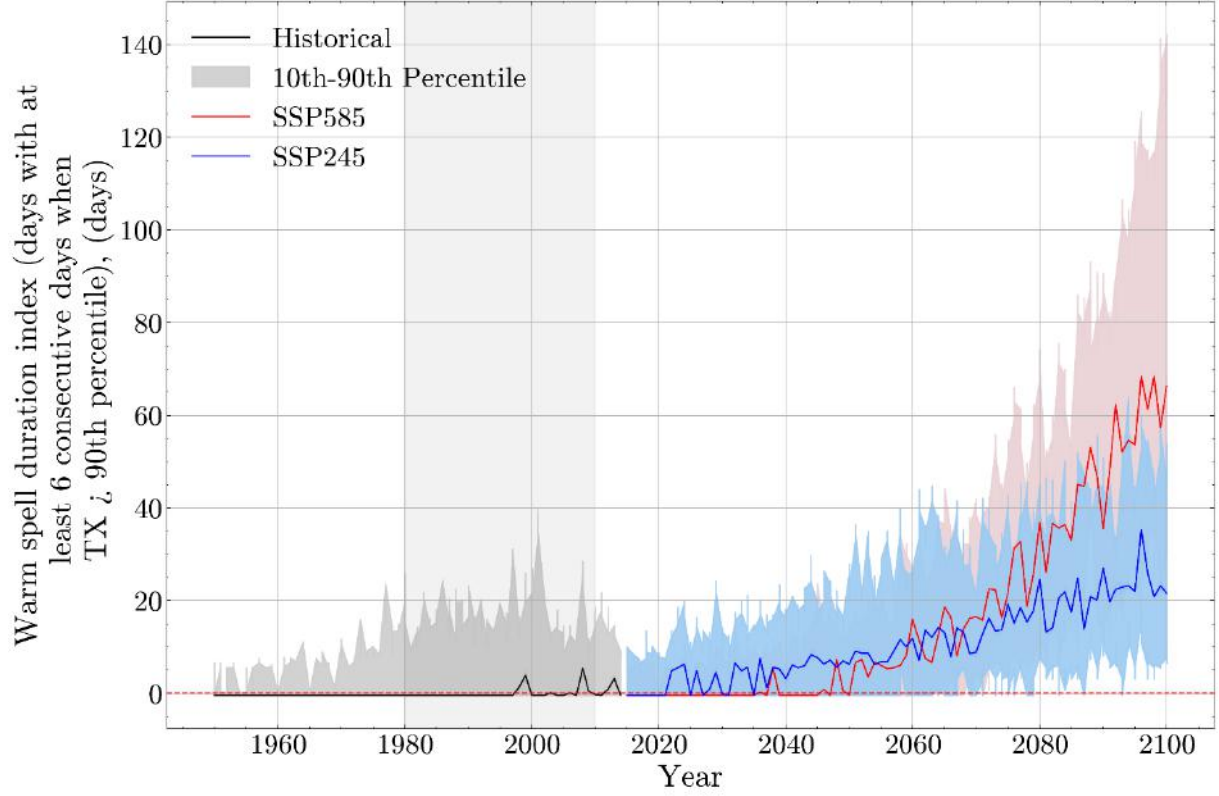
Şekil 5.10 Tarihsel ve Gelecek Dönemlerde SSP245 ve SSP585 Senaryoları İçin Sıcak Dönem Süresi İndisi
